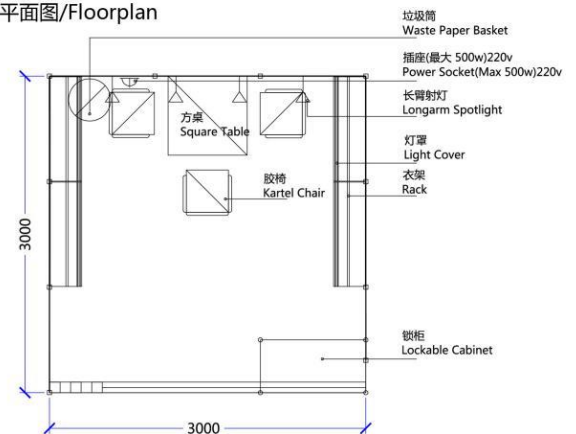
平面图/Floorplan
